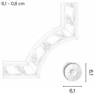
P20 + P101A Duropolymer® Ø 6,1 - 0,8 cm
